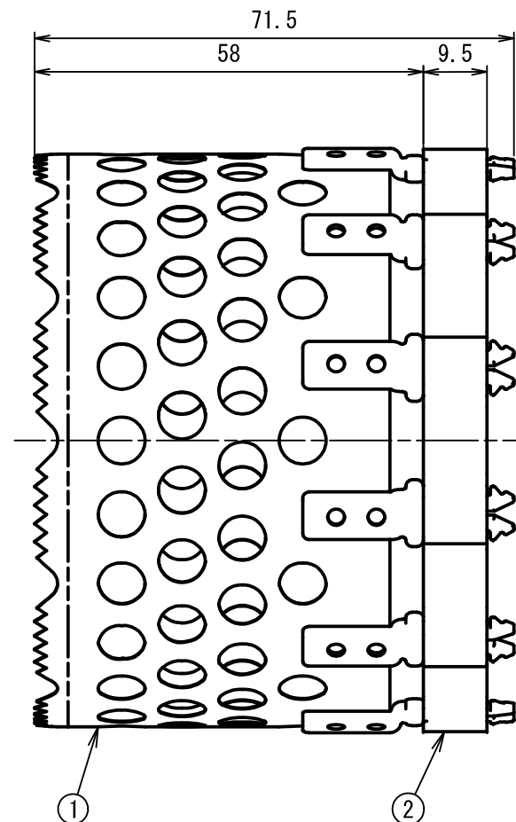
製品仕様図
